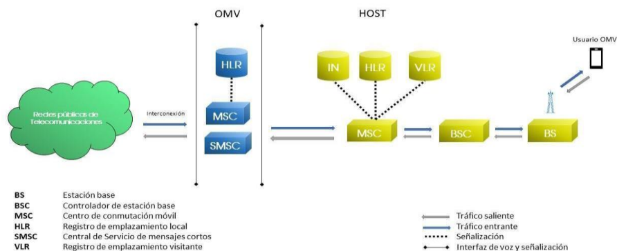
Diagrama 3. Flujo de tráfico de un OMV Completo/Agregador
