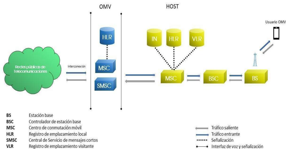
Diagrama 2. Flujo de tráfico de un OMV Completo/Agregador
