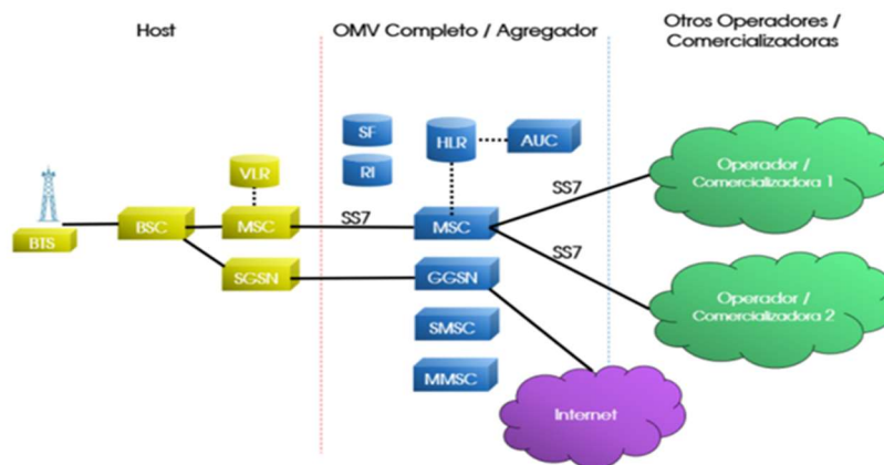
Diagrama 1. Elementos de la infraestructura de la red de un OMV Completo/Agregador
