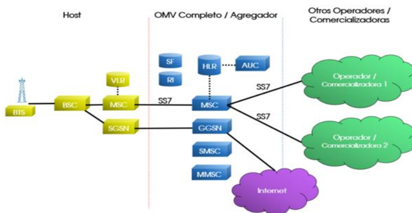
Diagrama 2 Elementos de la infraestructura de la red de un OMV Completo/Agregador
