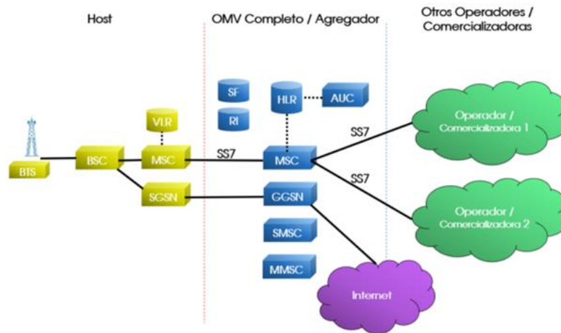
Diagrama 2 Elementos de la infraestructura de la red de un OMV Completo/Agredador
